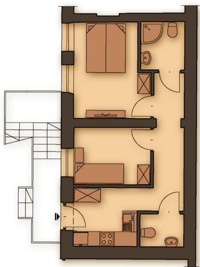
Rzut mieszkania
