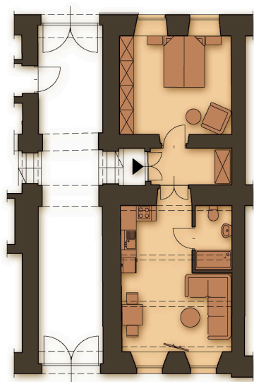
Rzut mieszkania
