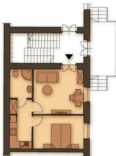
Rzut mieszkania
